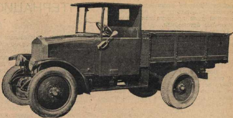
Полупортаторный грузовик завода „АМО“
